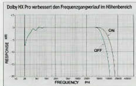
Dolby® HX Pro™ optimiert das Aufnahmepotential eines Decks im Höhenbereich, wodurch eine deutlich bessere Wiedergabe des hohen Frequenzbereichs ermöglicht wird.
