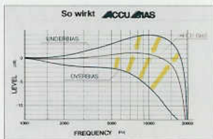
Das ONKYO Accubias-System bewirkt den bestmöglichen Frequenzgang für alle Ihre Cassetten, ungeachtet der Marke.
